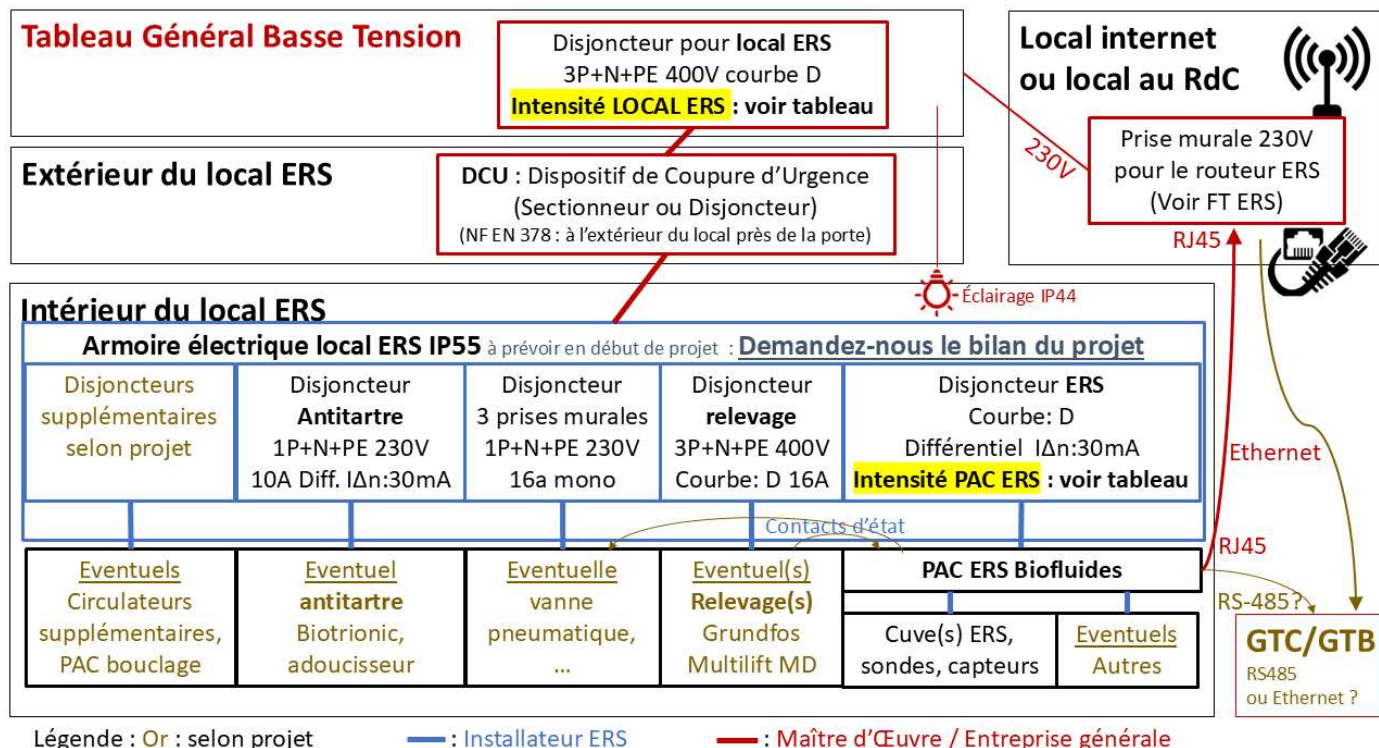
Figure 3: Illustration de l'alimentation électrique type
