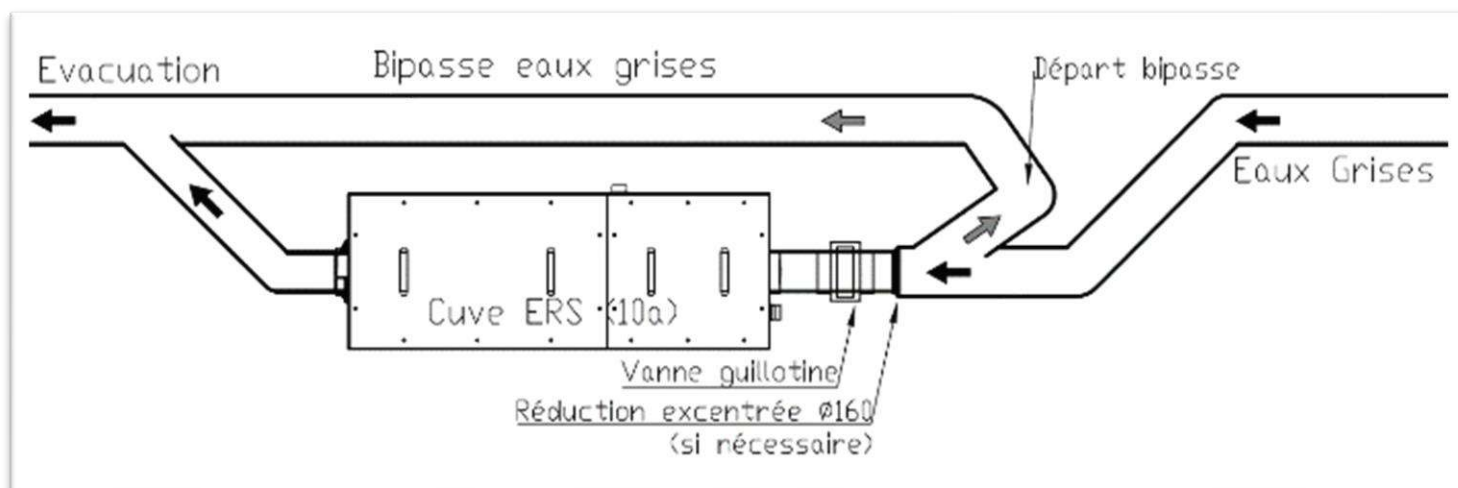
Figure 6 : Bypasse contournant la cuve - Vue du dessus
