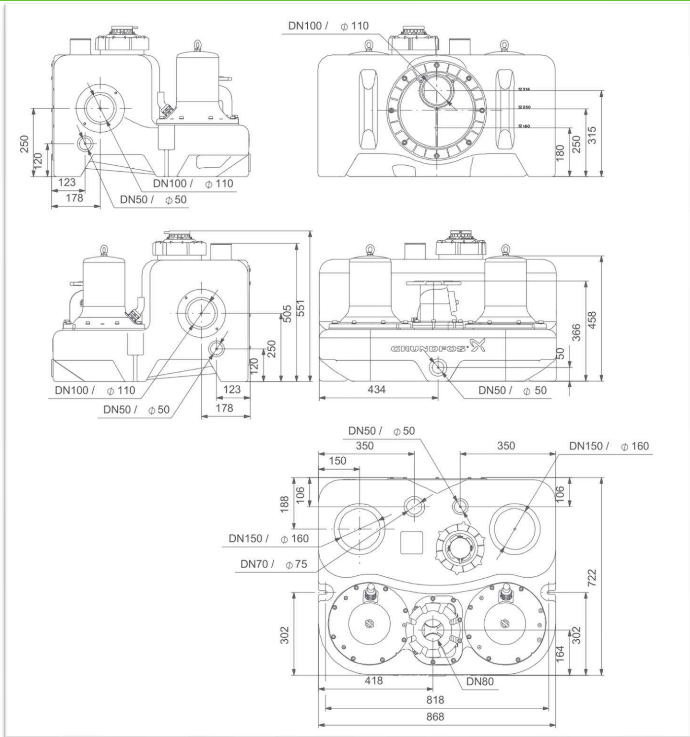
Figure 4 : exemple de dimension d'une Grundfos Multilift MD
