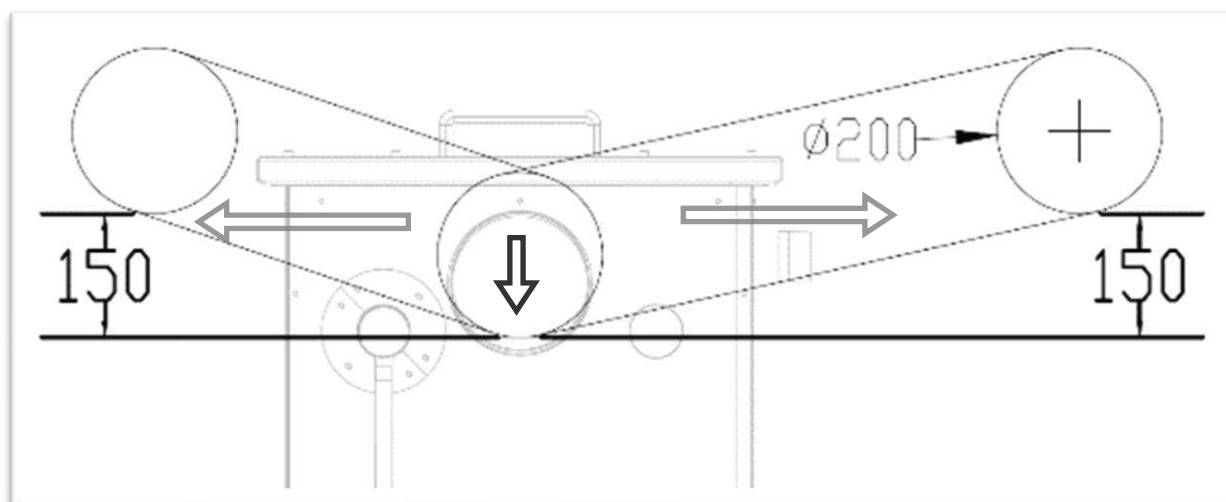
Figure 5 : Exemples de départ bypasse DN200 par rapport à la façade d'entrée eaux grises de cuve
